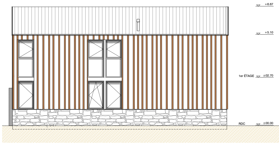
FAÇADE NORD
