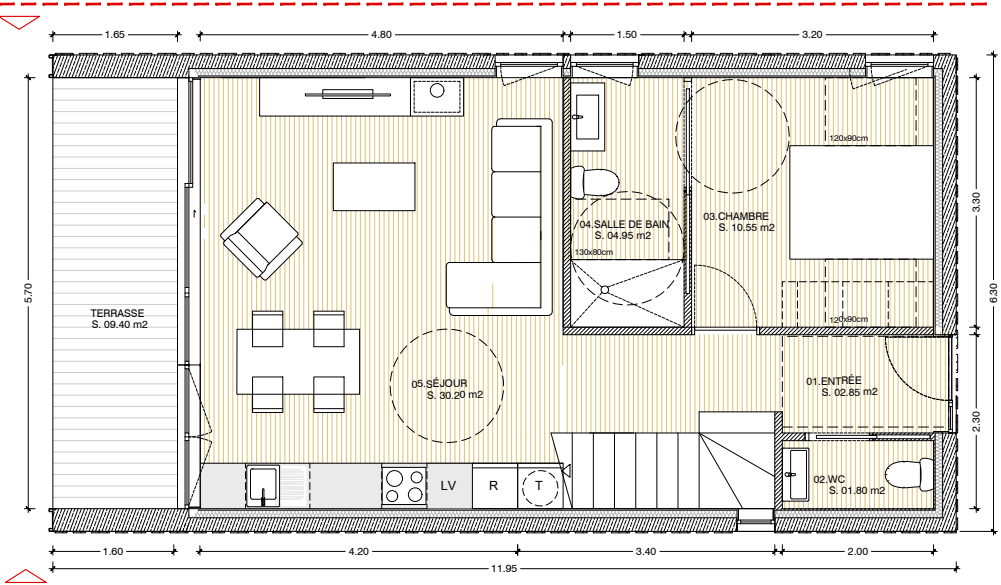
REZ-DE-CHAUSSÉE
