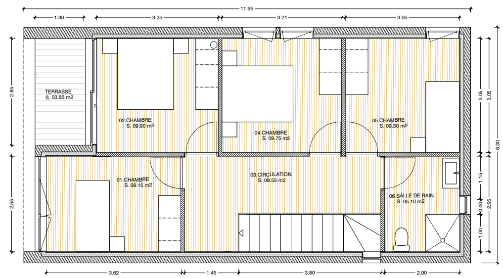
PREMIER ÉTAGE
