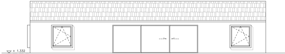
alçat sud
